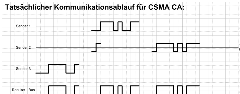
Abbildung 2: Aufgabe Kommunikation: CSMA/CA
