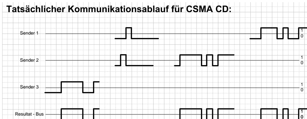
Abbildung 1: Aufgabe Kommunikation: CSMA/CD
